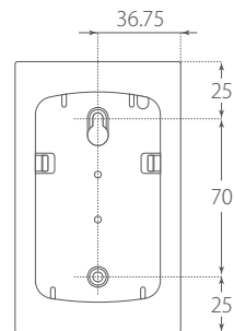
【ネジ穴位置】
