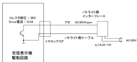
受信表示機 - パトライトIF説明図
