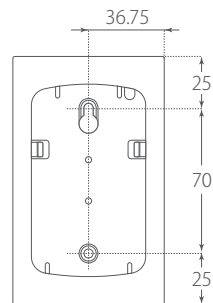
【ネジ穴位置】
